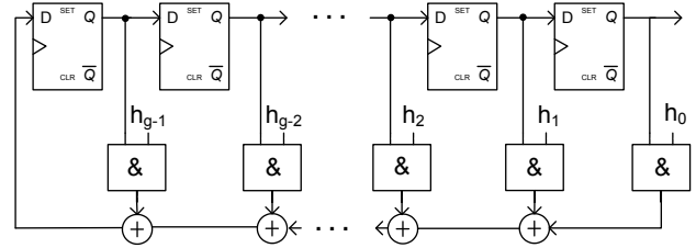
Fig. 2. Programmable LFSR [24].
